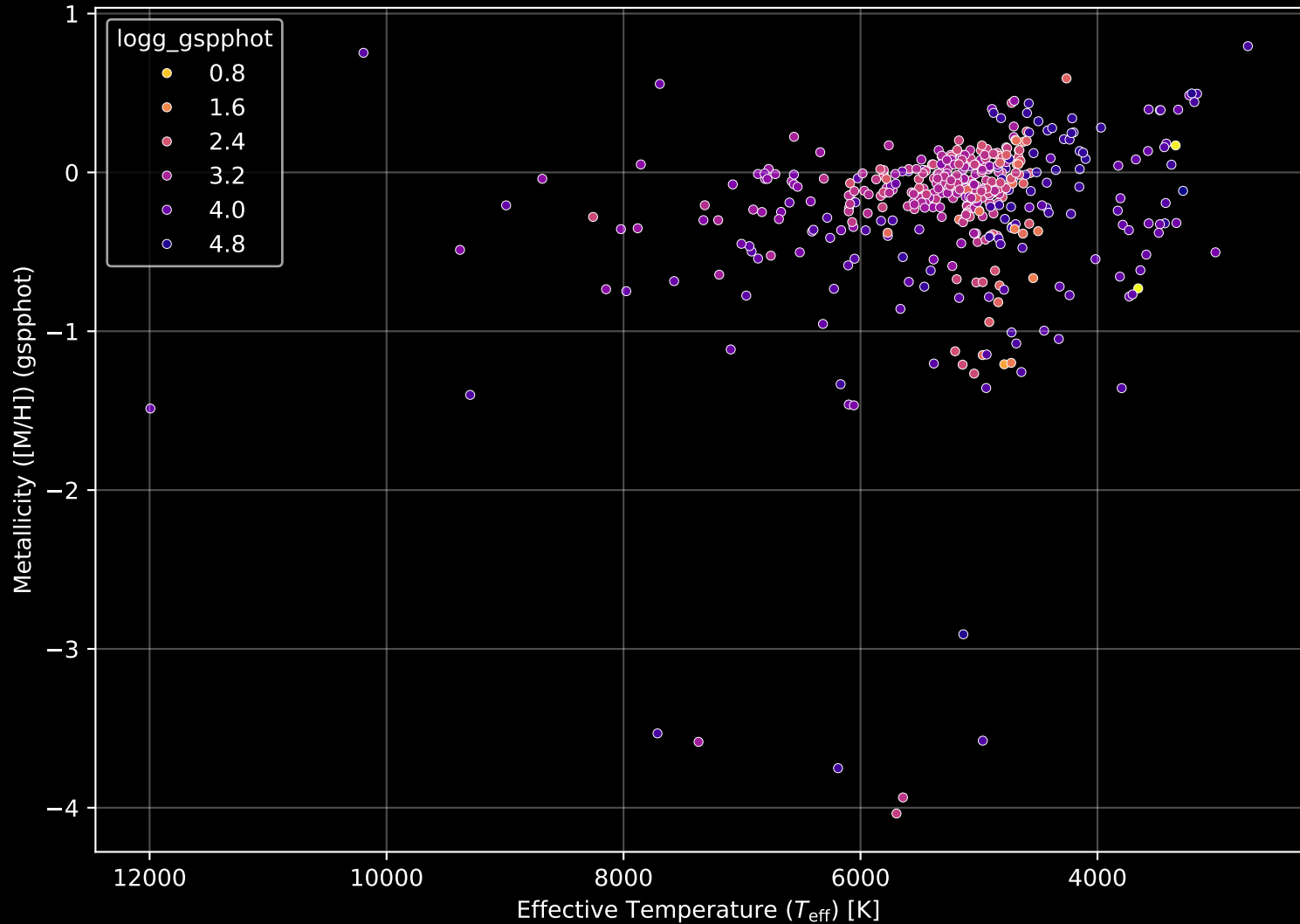
APOGEE DR17 Field: [N1333] Stellar Population Parameters (n= 442)
